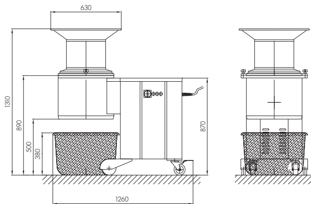
На чертеже CAD показана G 450
