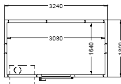
CRM/FRM 3240x1800 mm
