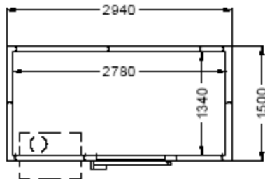
CRM/FRM 2940x1500 mm
