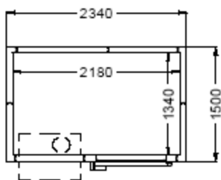
CRM/FRM 2340x1500 mm
